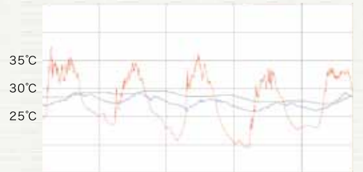
平成22年夏 猛暑の中の室温測定グラフ
